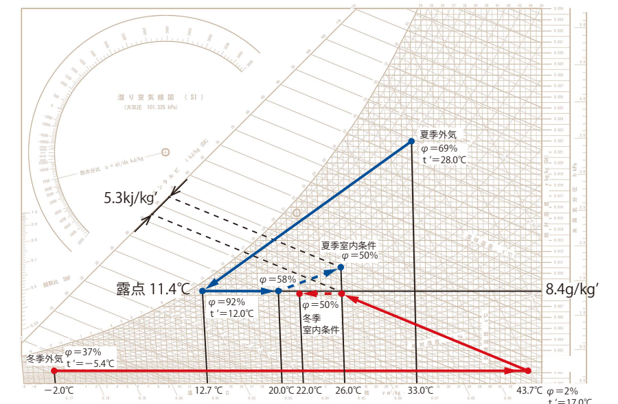
目標仕様空気線図
