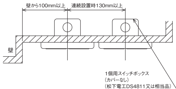
・ 取付要領図
